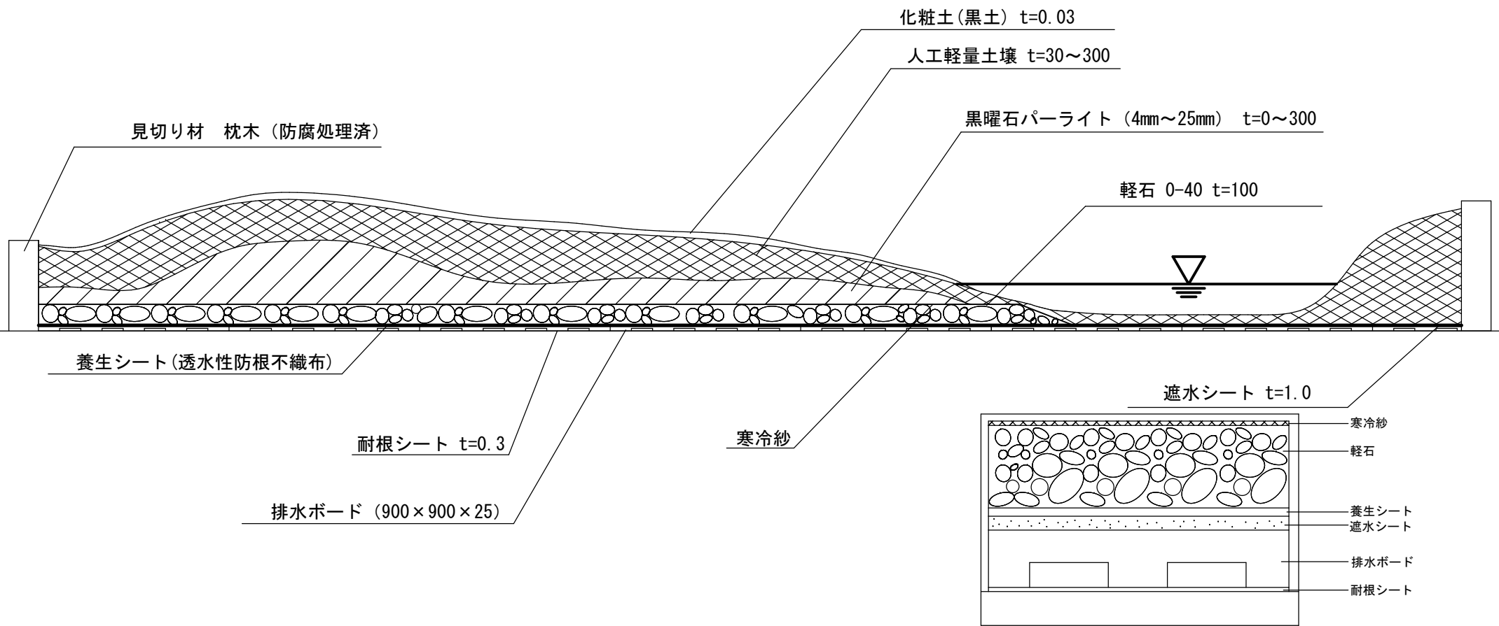
【標準断面図】
